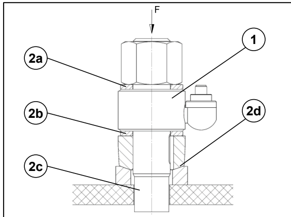
Rys. 2: Warunki instalacji
