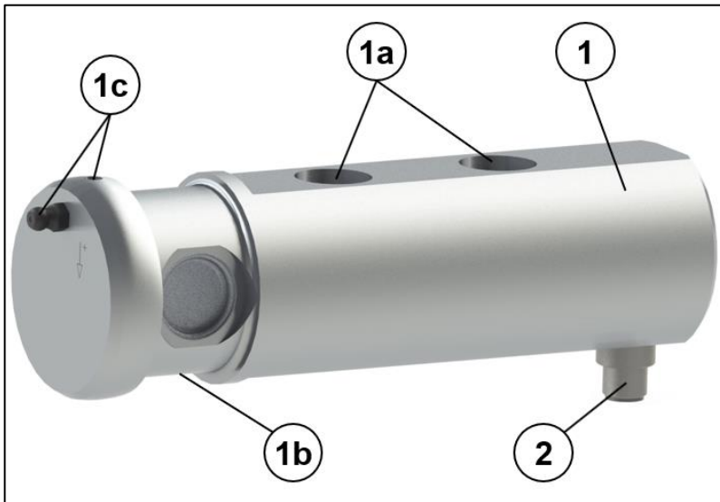
Afb. 1: Schuifkrachtsensor
