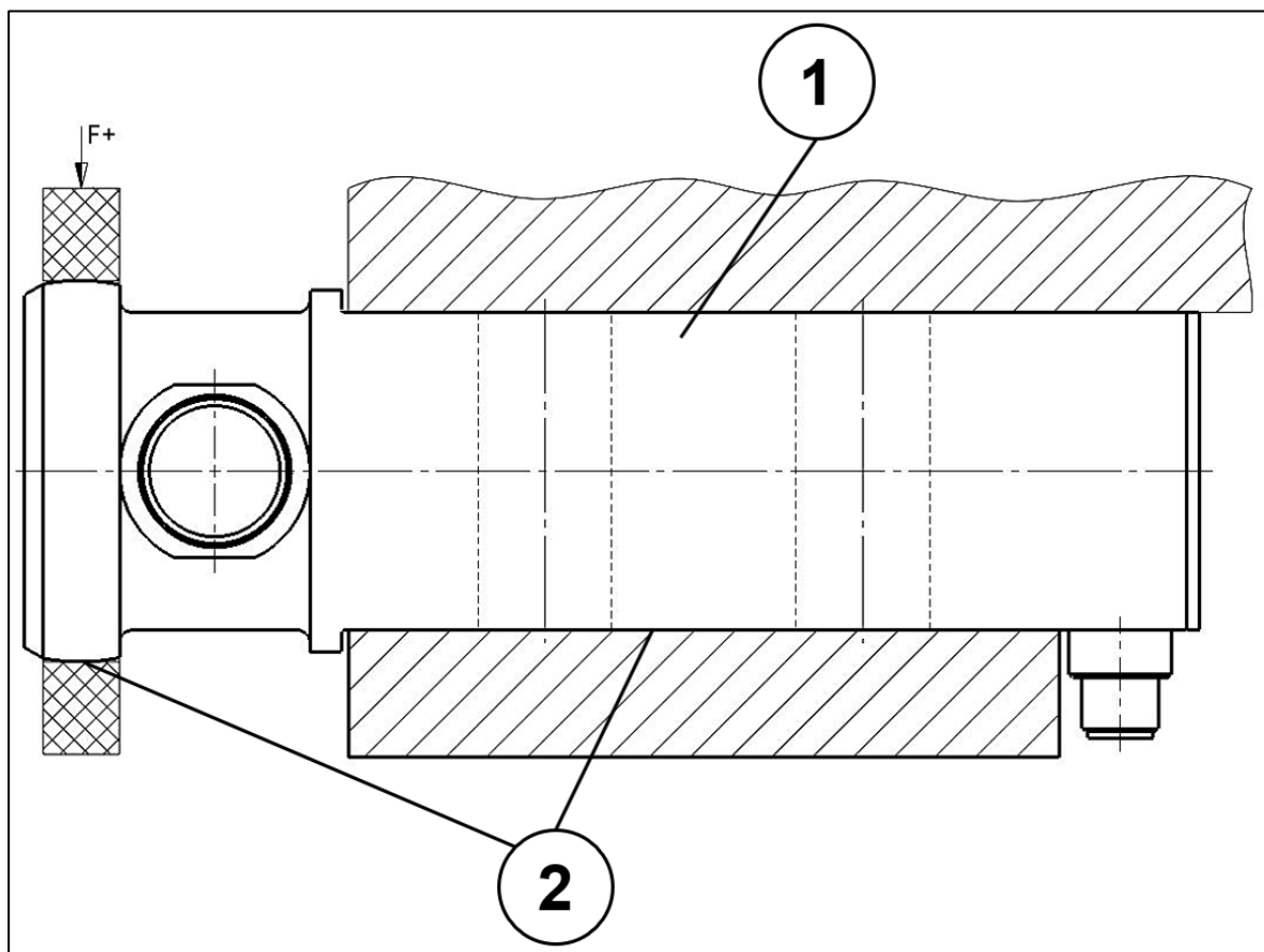
Afb. 2: Inbouwomstandigheden
