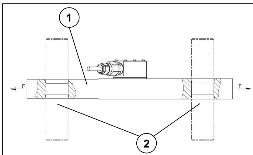
Afb. 2: Inbouwvoorwaarden
