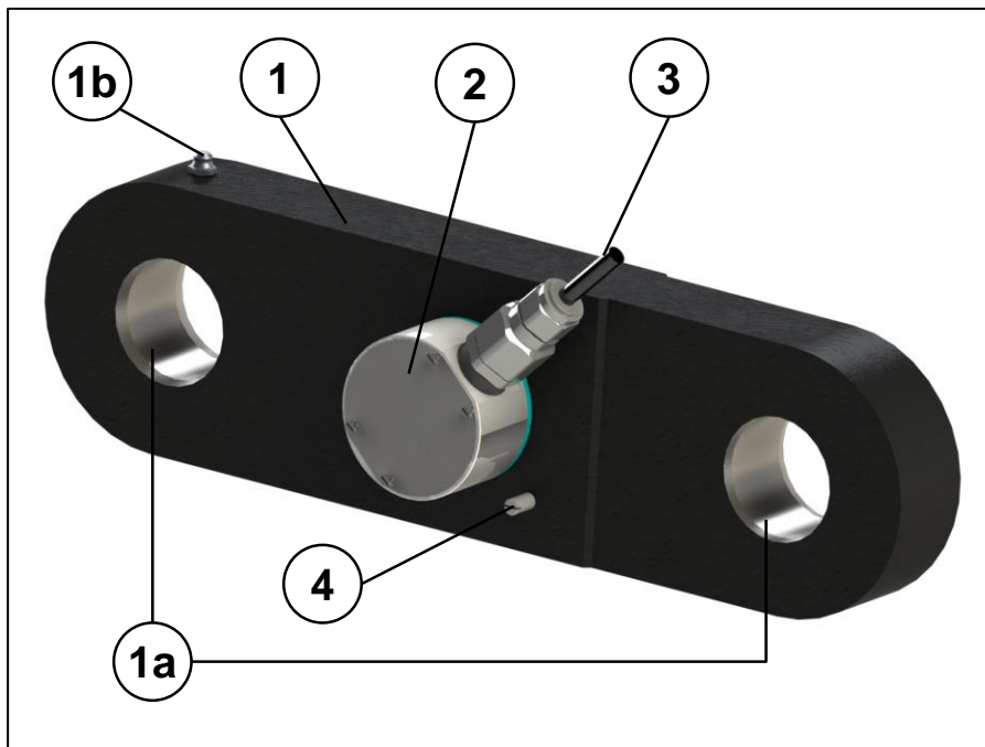
Image 1 : bride de mesure de force
