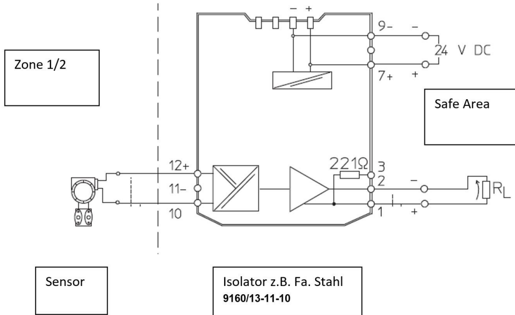
Kuva 6: Liitäntäesimerkki Anturi Ex i vahvistimella Ex DANGmicro2W***
