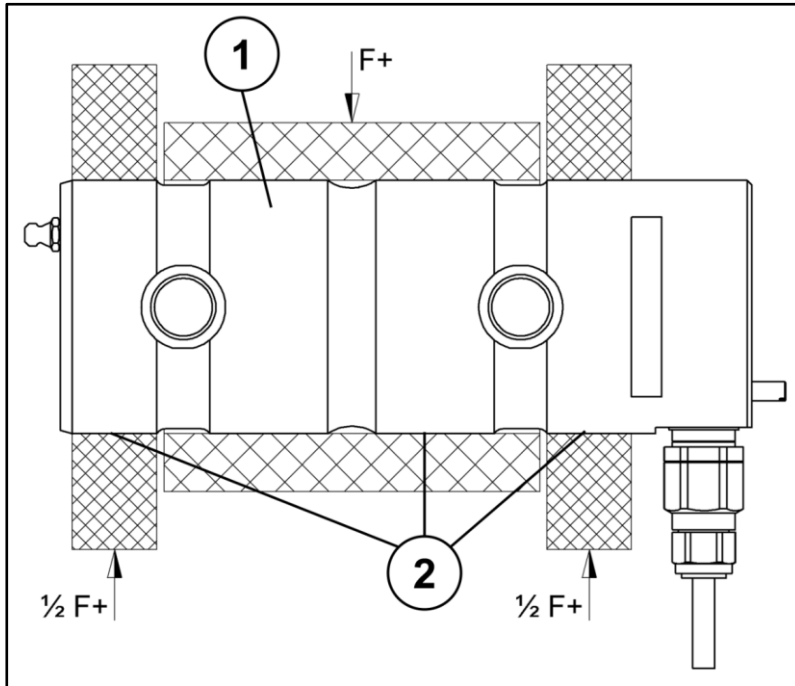
Kuva 2: Asennusolosuhteet
