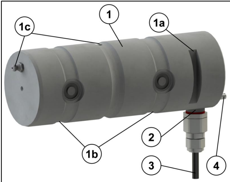
Kuva 1: Kuormituskenno
