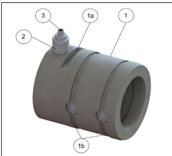
Bild 1: Kraftmesshülse
