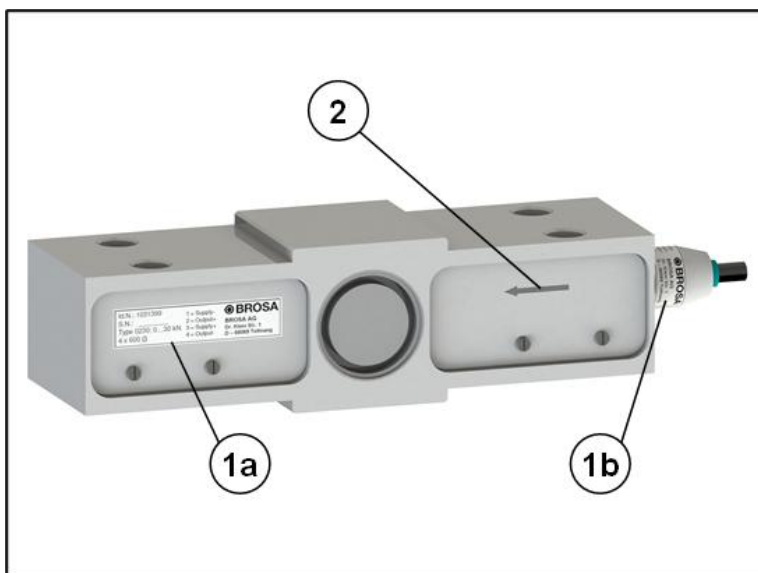
Bild 3: Messrichtung
