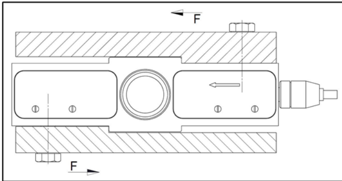
Bild 2: Einbauverhältnisse
