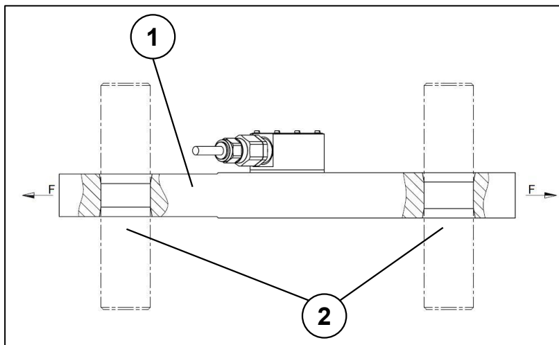
Bild 2: Einbauverhältnisse
