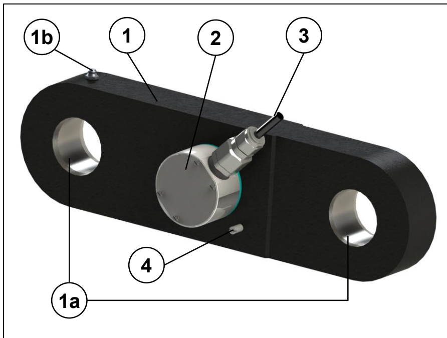
Bild 1: Kraftmesslasche
