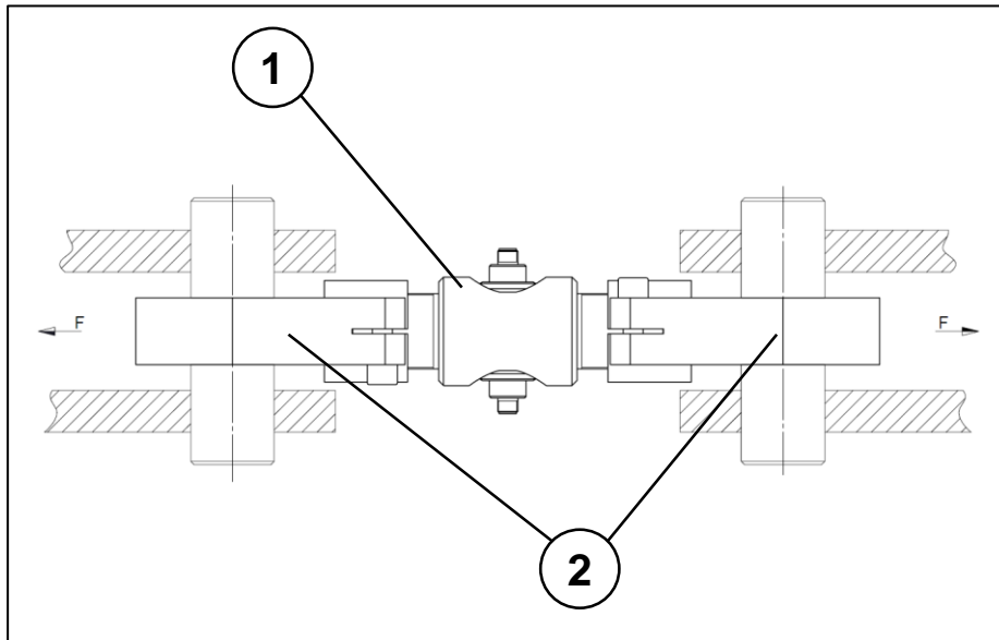
Bild 2: Einbauverhältnisse
