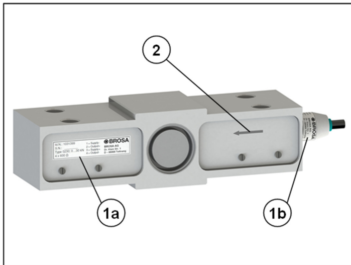
Bild 3: Kennzeichnung des Kraftmessblocks
