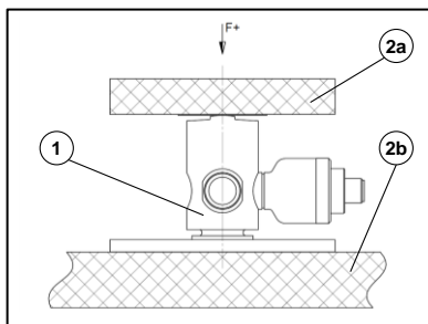
Bild 2: Einbauverhältnisse
